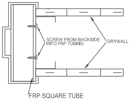
FRP SQUARE TUBE DRYWALL STUD ANCHOR
